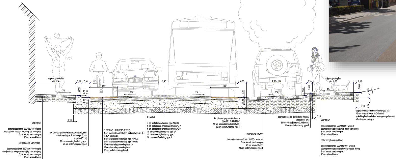
TYPEDWARSPROFIEL FABRIEKSTRAAT schaal 1/25
