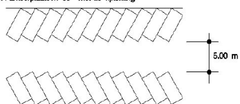
Figuur 4. Parkeerplaatsen 60° met de rijrichting
